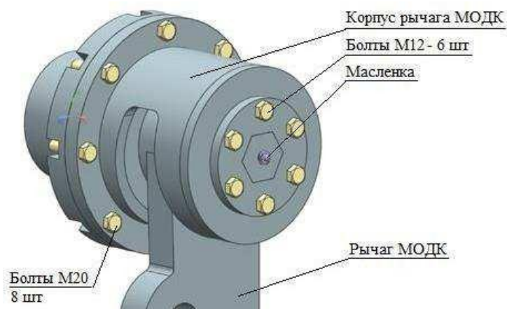
2-сурет - Рычаг пен МОДК корпусының үлкейтілген көрінісі
