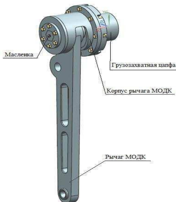
1-сурет – Рычаг пен МОДК корпусының жалпы көрінісі
