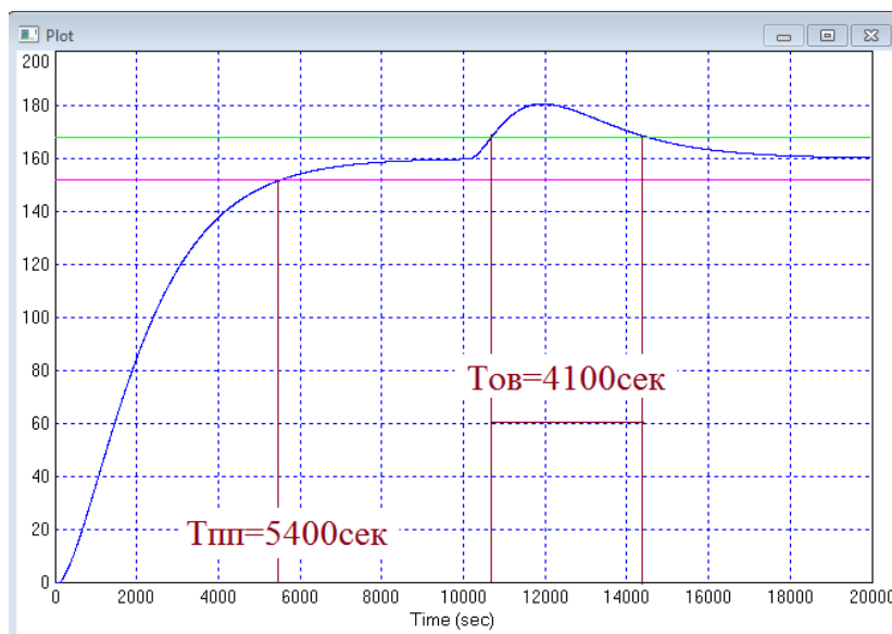
Рисунок 6 – Определение показателей качества переходного процесса
