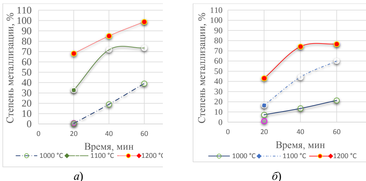
Рисунок 3 – Зависимость степени восстановления железосодержащего порошка от температуры без добавления жидкого стекла ( а ), с добавлением 15% жидкого стекла ( б ).
