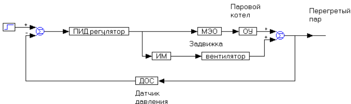
Рисунок 2 – Схема системы автоматического регулирования давления пара на выходе из парового котла
