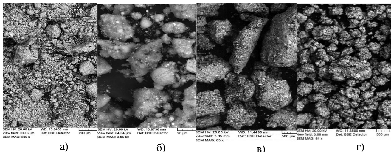
Рисунок 2 – Микроструктура обогащенной аспирационной пыли сталеплавильных дуговых печей: а – пыль при 200-кратном увеличении; б – пыль при увеличении в 3000 раз; в - с добавлением 5% ЖС с размером фракций 1 - 0,315 мм; г - 15% ЖС с размером фракций 0,63 - 0,2 мм
