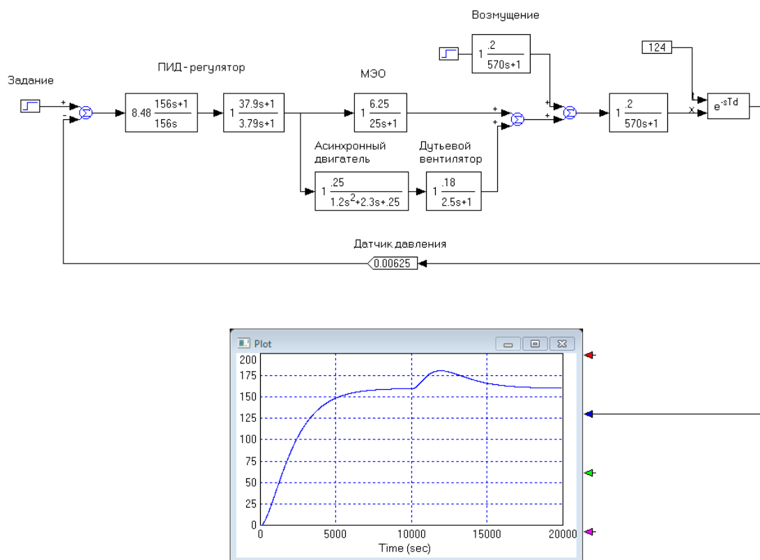
Рисунок 5 – Схема модели САР давления пара на выходе котла с ПИД–алгоритмом управления
