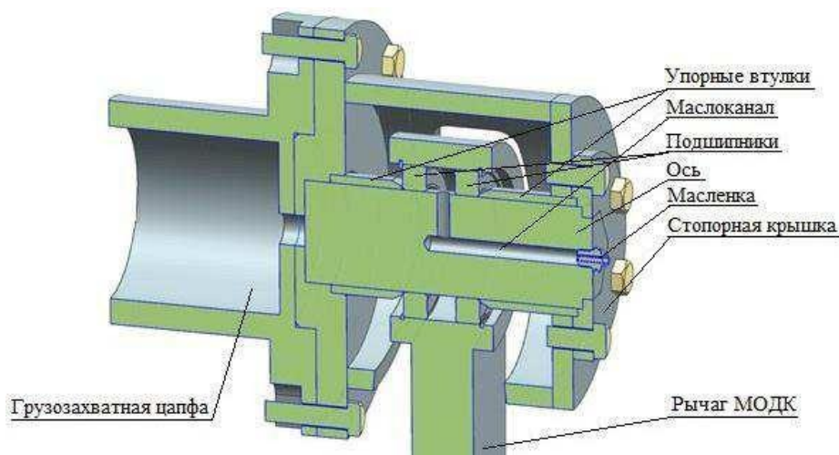
3-сурет – МОДК рычагының және корпусының секциялық көрінісі
