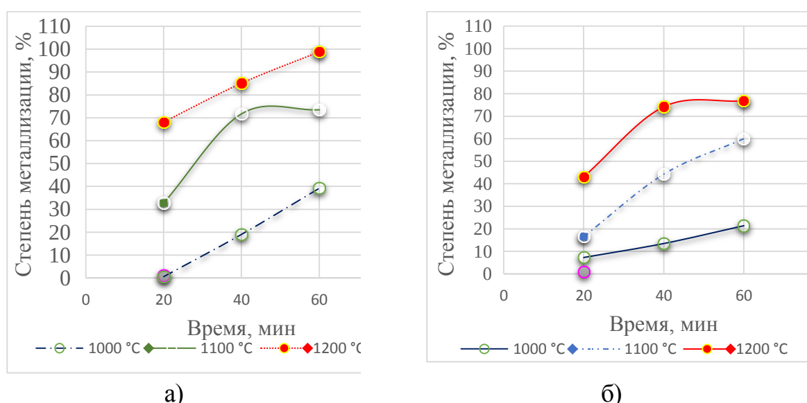
Рисунок 3 – Зависимость степени восстановления железосодержащего тонкодисперсного порошка от температуры без добавления жидкого стекла (а), с добавлением 15% жидкого стекла (б).
