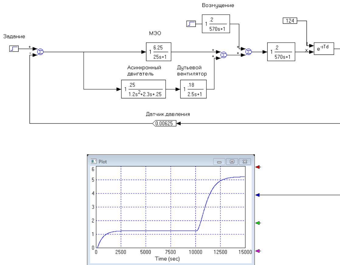
Рисунок 4 – Переходная характеристика САР давления пара
