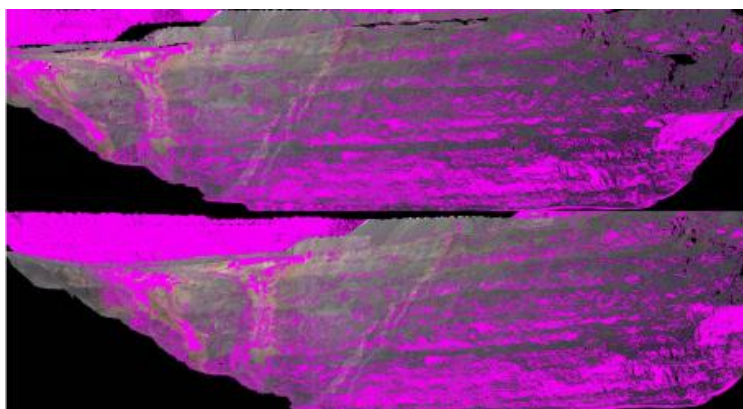
Рисунок 3 - Наложения двух сканов северо-западного участка борта карьера март-октябрь
