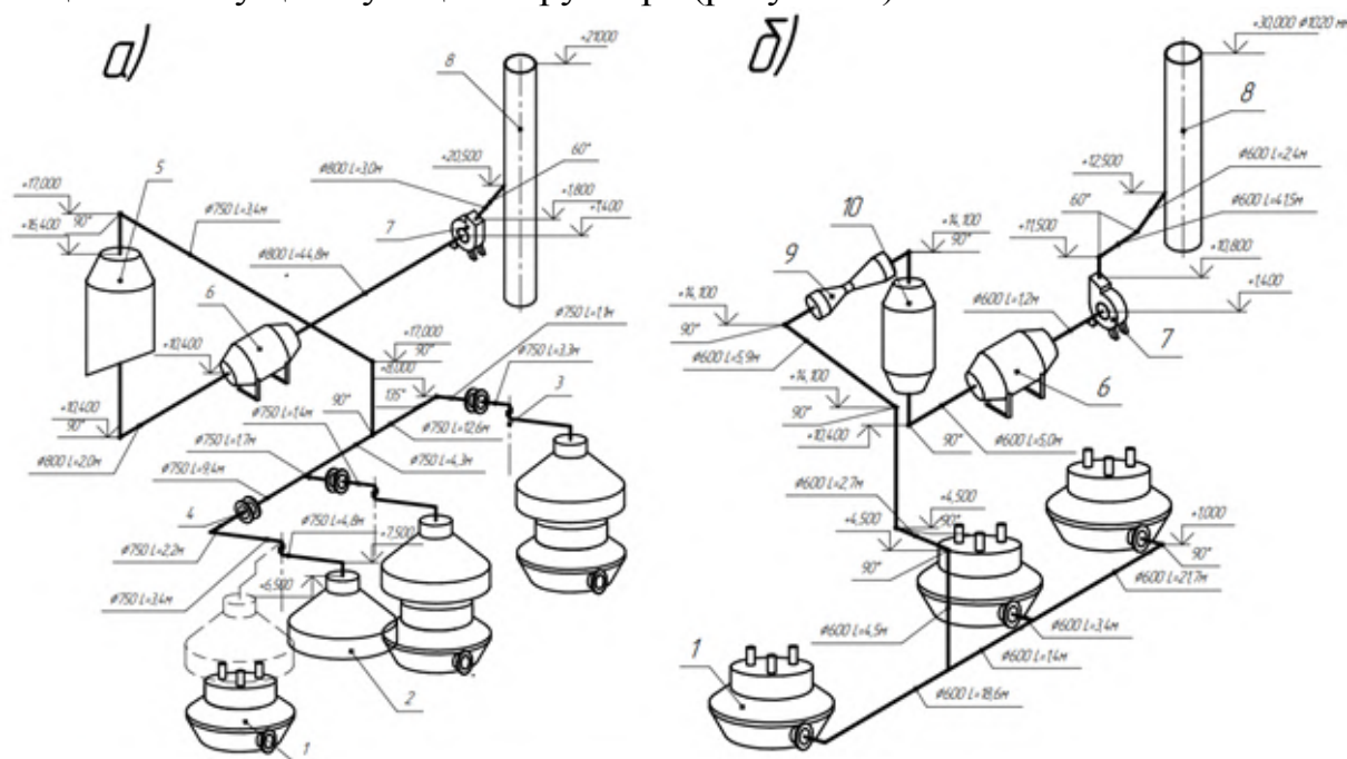
а – очистка газов от зонтов ДСП; б – очистка газов, отбираемых от корпуса печей:
