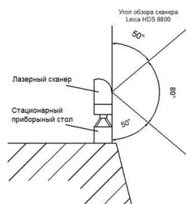
Рисунок 2 -Угол обзора сканера
