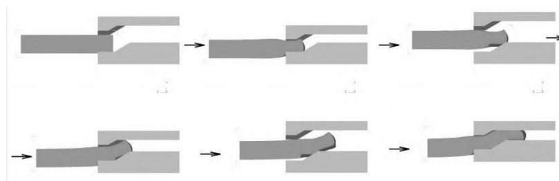
Рисунок 3 - Схема деформирования заготовок в ступенчато-клиновидных бойках
