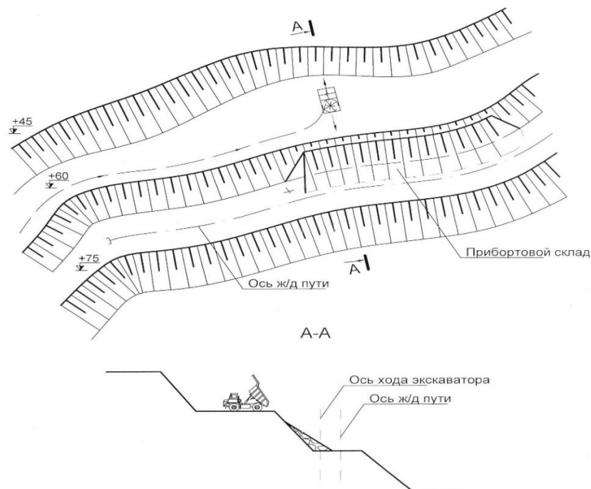
Рисунок 3 - Приступный внутрикарьерный перегрузочный склад
