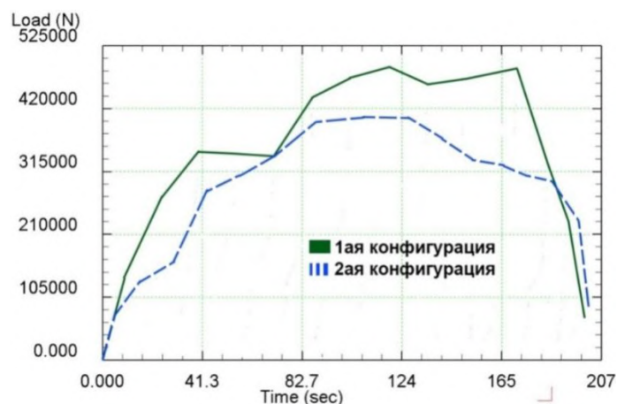
Рисунок 1 – Значения усилий при протяжке в ступенчато-клиновидных бойках
