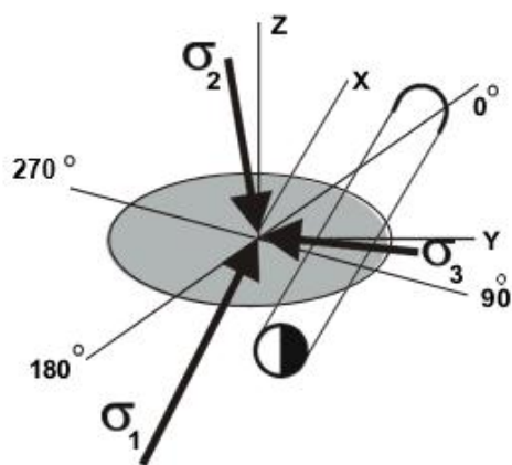
Рисунок 2 –Ориентировка компонент тензора напряжений в массиве шахты «Молодежная» относительно направления проведения ортов
