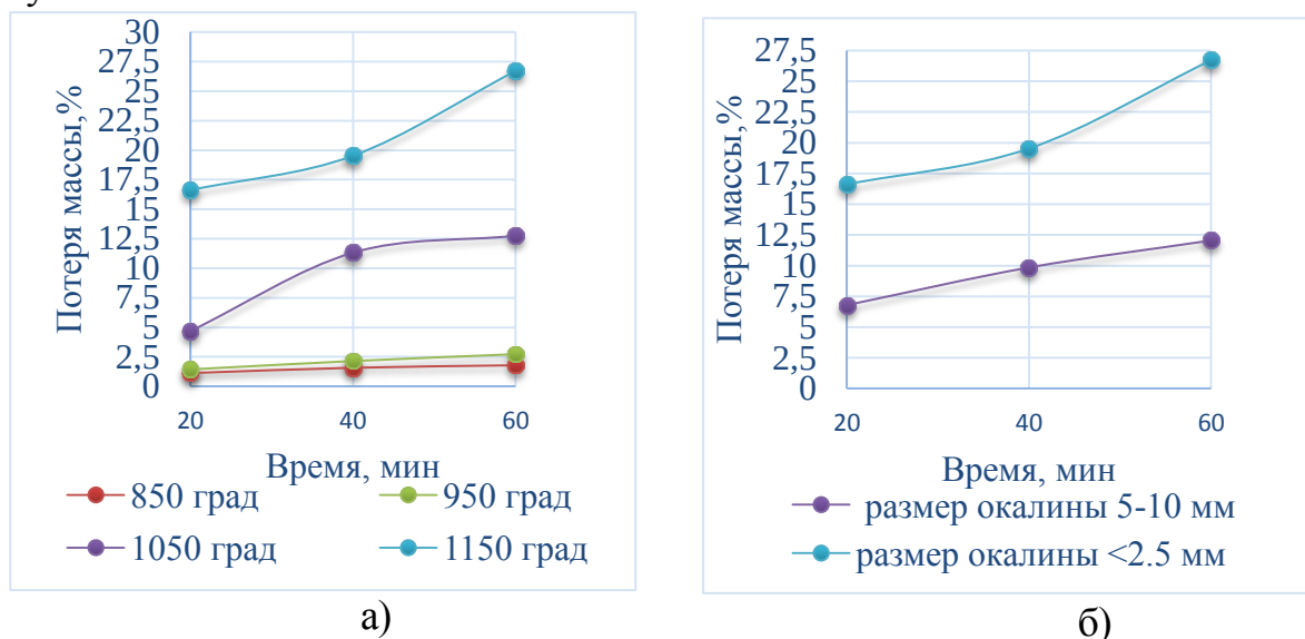
Рисунок 1 – Зависимость степени восстановления окалины от температуры (а) и размера частиц при температуре 1050°C (б)
