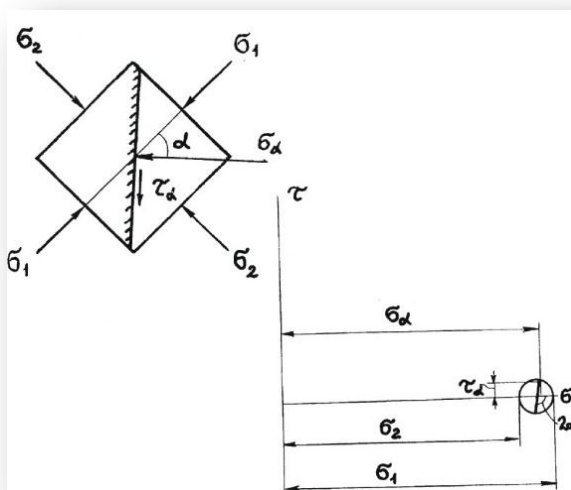
Рисунок 1 Напряженное состояние массива в плоскости нормальной к оси штрека шахты «Молодежная» ДГОК и круг Мора, построенные на квази главных напряжениях и соответствующий наиболее опасной системе трещин
