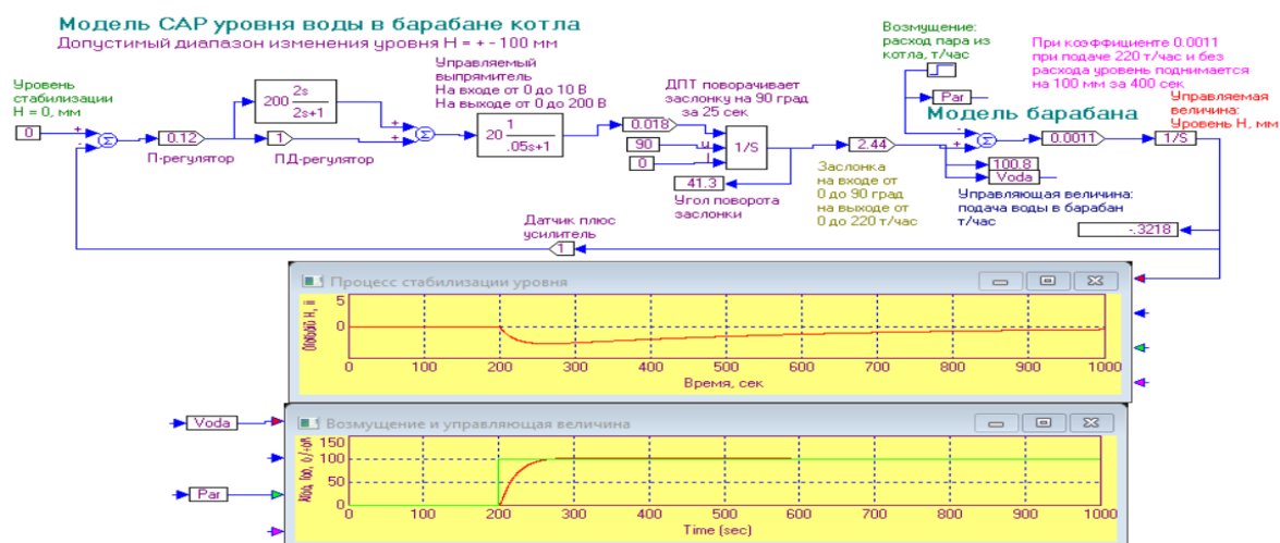
Рисунок 1 – Модель САУ уровня воды
