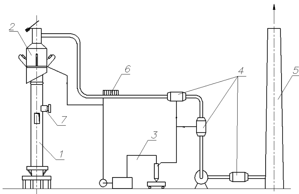
Рисунок 1– Схема ваграночной установки с многоступенчатой системой очистки с применением конденсационного пылеосаждения: 1 – вагранка; 2 – мокрый пылеуловитель – полый скруббер; 3 – система очистки и подачи воды; 4 – каплеуловители горизонтальный и вертикальный; 5 – дымовая труба; 6 – форсунки; 7 – узел дожигания СО
