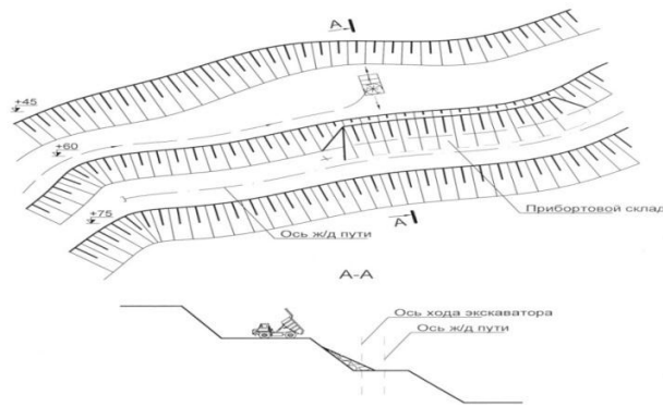
Рисунок 1 - Приуступный внутрикарьерный перегрузочный склад
