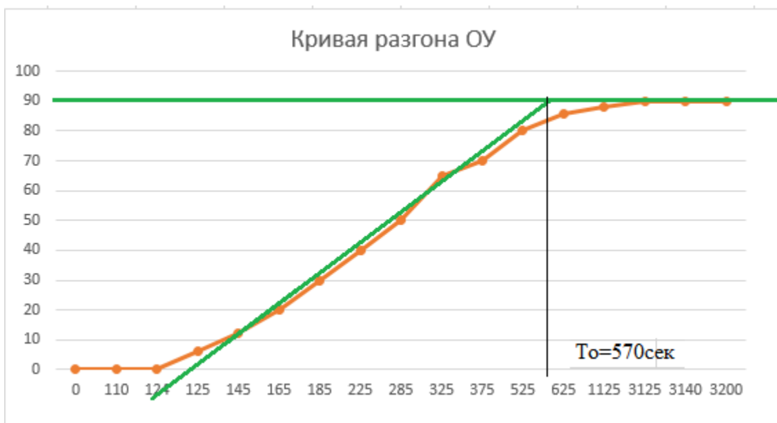
Рисунок 3 – Кривая разгона парового котла
